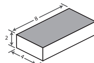
MORTARLESS PAVER
